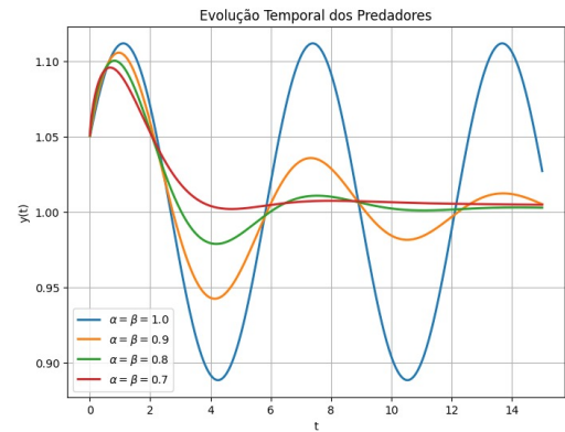
(b) Predadores y(t) .
