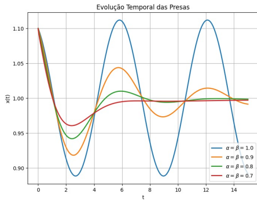
(a) Presas x(t) .
