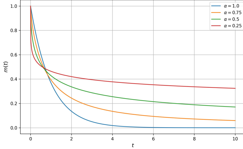
Fig. 1: Solução m(t) = m_0 E_\alpha(-kt^\alpha) para diferentes \alpha .
