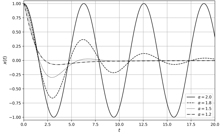
Fig. 2: Solução x(t) = x_0 E_\alpha(-\omega^2 t^\alpha) para \alpha \in (1, 2] . O amortecimento intrínseco intensifica-se conforme \alpha se afasta de 2.
