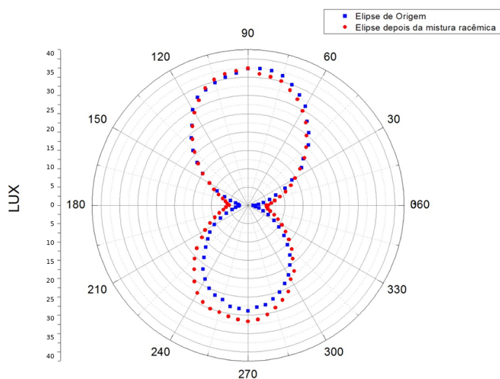
Fig. 3. Elipses de polarização, em gráfico polar, da cela sem e com mistura racêmica do limoneno.
