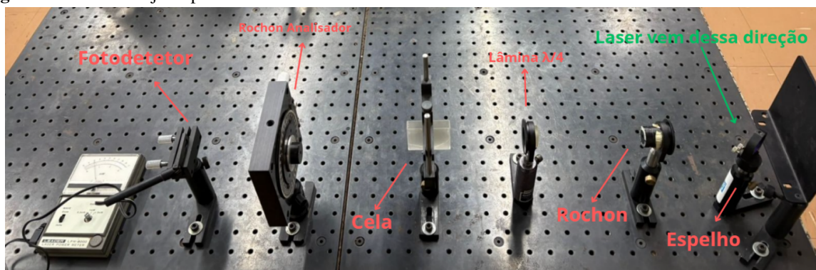
Fig. 1. Parte do arranjo experimental.
