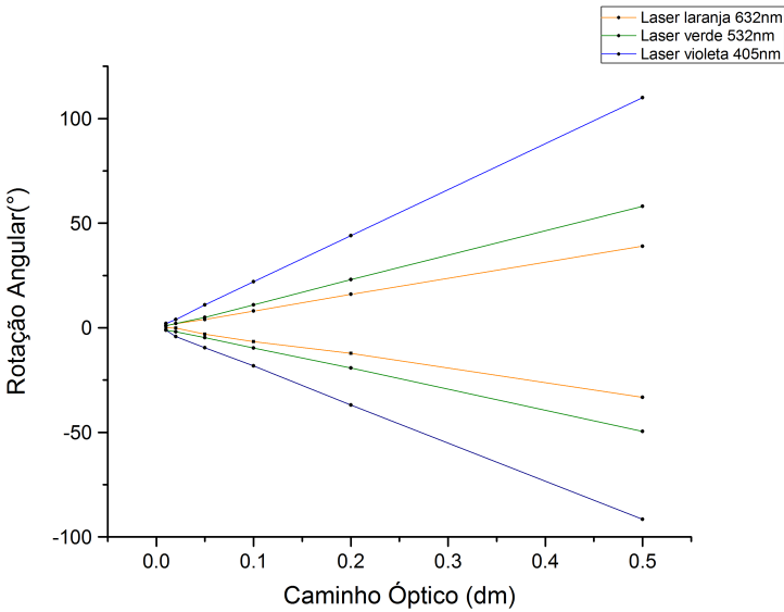
Fig. 2. Rotação óptica em função do caminho óptico para os enantiômeros do limoneno nos três comprimentos de onda investigados.
