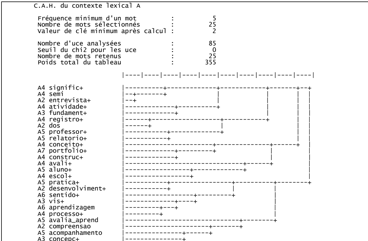
Figura 5 - Classificação Hierárquica Ascendente, elementos intraclasses
