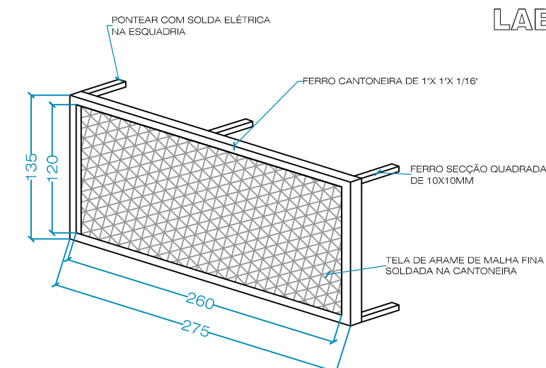
DETALHE - TELAS PARA JANELAS Escala 1 : 100
