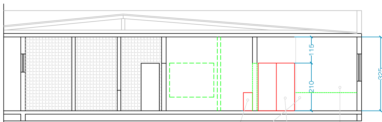
CORTE A - B LAVATÓRIO A SER REALOCADO ESC. 1:100
