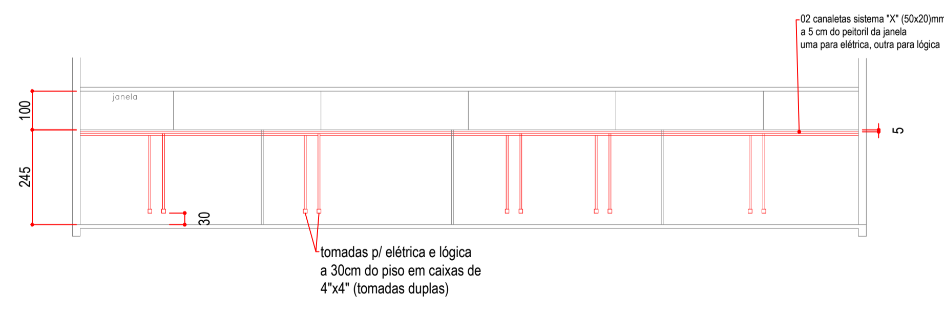
DETALHE 1 DAS CANALETAS SOB O PEITORIL DA JANELA escala: 1:100
